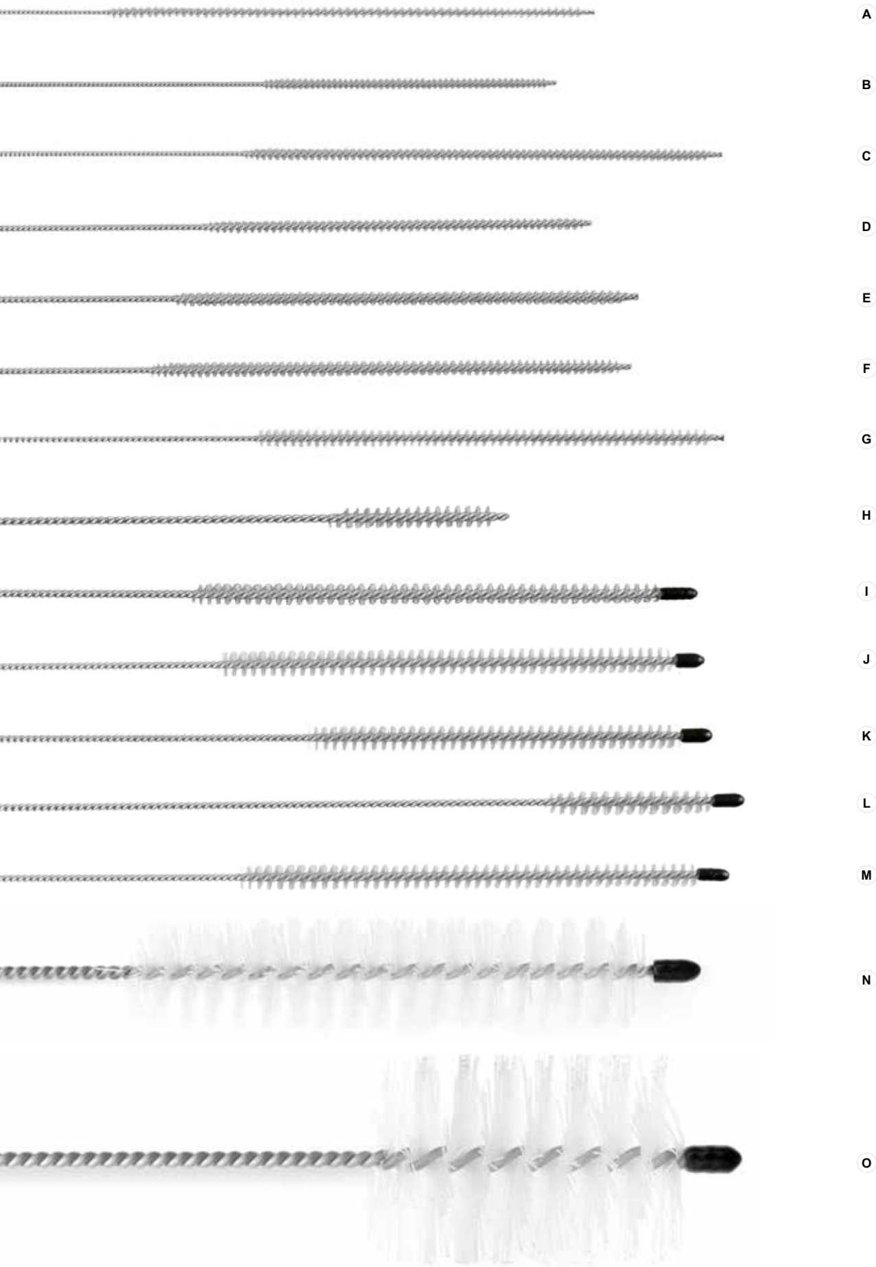
BRUSH TIP DETAILS SHOWN ACTUAL SIZE
